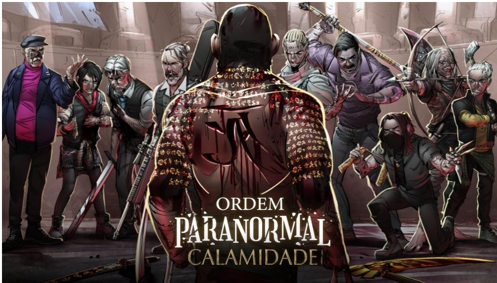
Figura 4 - Quarta Campanha
